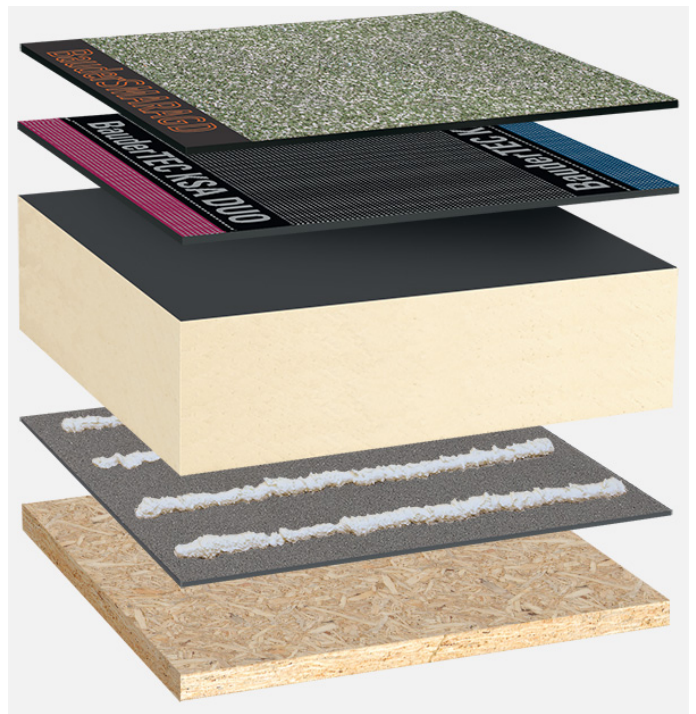
Sustav: HG_PIR-FA_S_01
